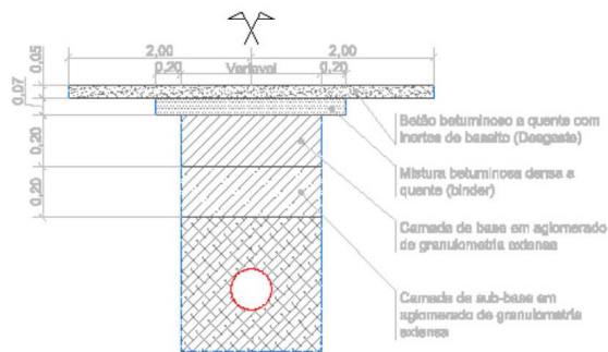
Sentido longitudinal ao eixo da rua
