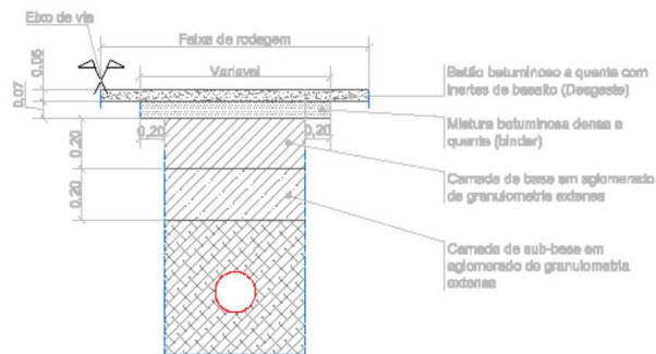
Sentido longitudinal ao eixo da rua
